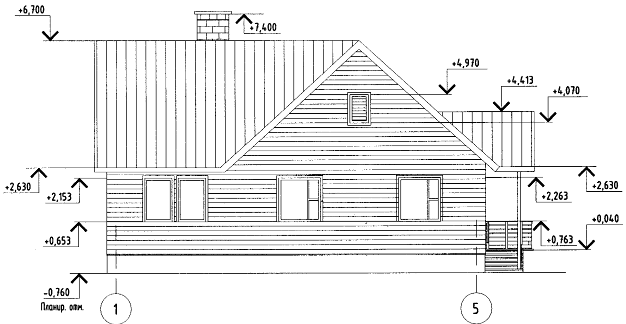
Фасад 1 - 5
